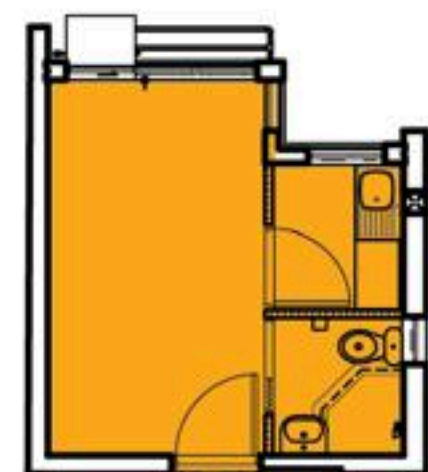
A 型單位 / 1-2 人 (6 及 25 號單位) 14.05 平方米
