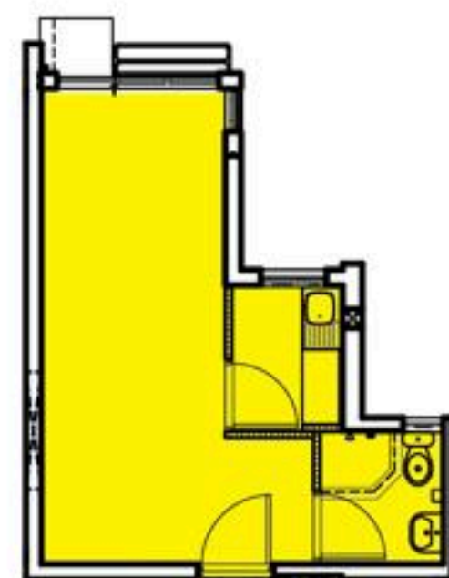
B 型單位 / 2-3 人 (1、7、10、11、14-16、 17、20 及 22-24 號單位) 21.49 平方米
